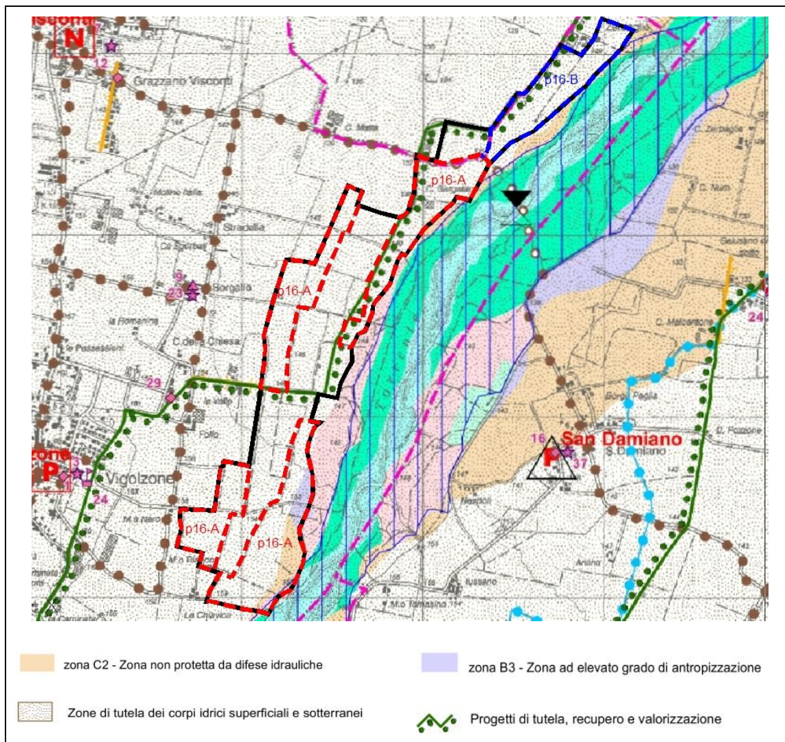
Fig. 2.1.1 - Stralcio della Tav. A1.5 del PTCP di Piacenza - Tutela Ambientale, storica e paesaggistica
